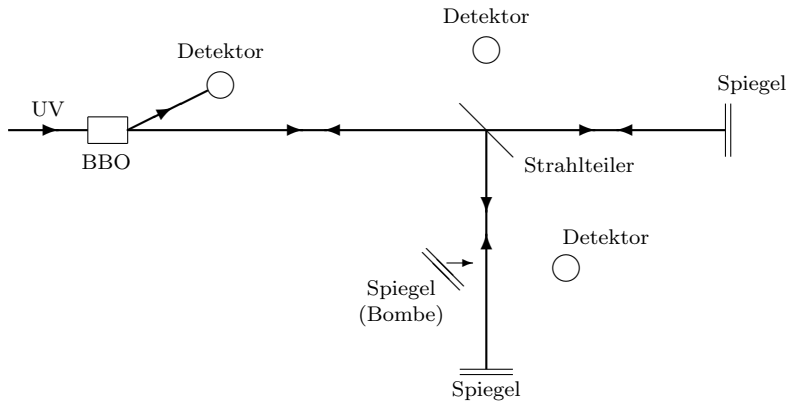
Abbildung 5: Experimentelle Realisierung des „Knallerexperiments“ in einem Michelson-Interferometer. In einem BBO-Kristall werden zwei Photonen erzeugt, von denen eines nachgewiesen wird. Dadurch ist bekannt, dass sich ein zweites Photon in der experimentellen Anordnung befindet. Der bewegliche Spiegel („Bombe“) kann nach rechts in den Strahlengang geschoben werden und lenkt das Photon auf den Detektor. Der obere Detektor (dunkel) sollte nur Ereignisse anzeigen, bei denen ein Hindernis im zweiten Strahlengang vorhanden ist. Der untere Detektor zeigt an, ob das Hindernis getroffen wurde.
