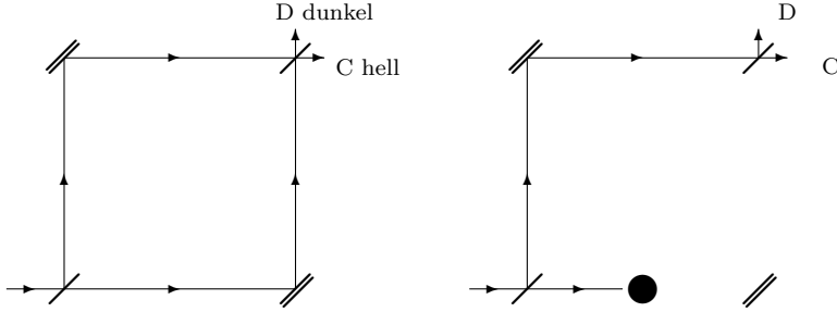
Abbildung 4: Mach-Zehnder Interferometer ohne und mit Hindernis in einem Strahlengang. Ohne Hindernis sollte der Detektor bei D nie ansprechen, mit Hindernis in rund einem Viertel der Fälle.
