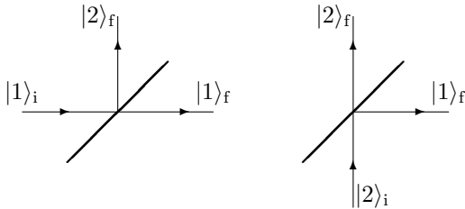
Abbildung 1: Die beiden Strahlengänge in einem Strahlteiler in Abhängigkeit vom Anfangszustand. Ordnet man jeder Reflexion einen Faktor i zu, erhält man die Matrix in Gl. 2.
