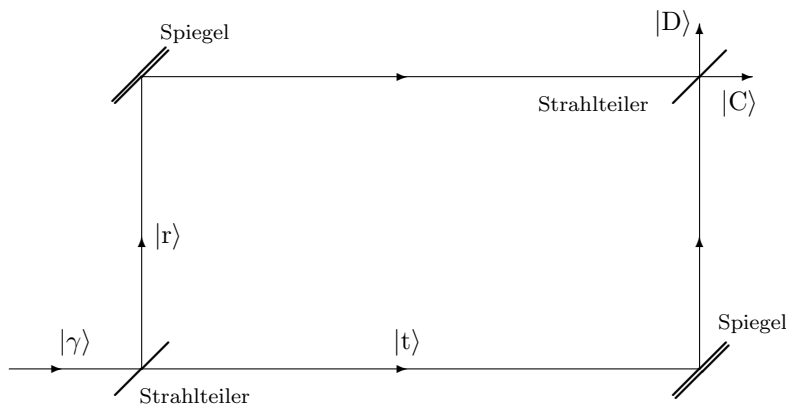
Abbildung 2: Mach-Zehnder-Interferometer. Der Strahl trifft auf einen ersten Strahlteiler. Die beiden Teilstrahlen r und t werden von Spiegeln auf einen zweiten Strahlteiler gelenkt, hinter dem es zu konstruktiver bzw. destruktiver Interferenz kommen kann.
