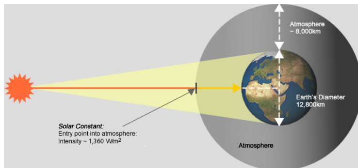
Abbildung 1: Definition der Solarkonstanten. Die gemessene Intensität der Sonnenstrahlung oberhalb der Erdatmosphäre wird auf den mittleren Abstand Sonne-Erde umgerechnet. (aus [1])
