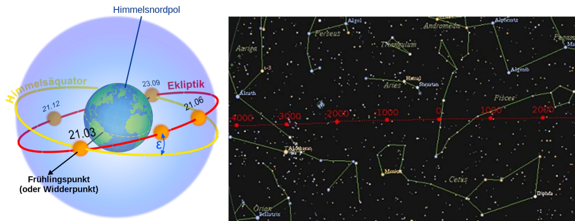
Abbildung 1.1: (links) Der Frühlingspunkt als der Schnittpunkt zwischen dem Himmelsäquator und der Ekliptik. (rechts) Der Frühlingspunkt in den letzten Jahrtausenden. Während der Frühlingspunkt heute (im Jahr 2023) im Sternbild Fische (Pisces) steht, stand er vor rund 2500 Jahren im Sternbild Widder (Aries). Und in einigen Jahrhunderten wird er im Sternbild Wassermann stehen. (links [4], rechts [2])
