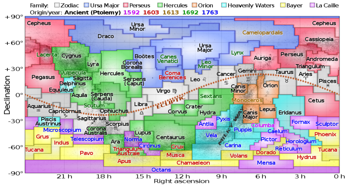
Abbildung 1.2: Die 88 Sternbilder in der Äquatorialdarstellung. Die Hintergrundfarben beziehen sich auf verschiedene Gruppen von Sternbildern, insbesondere handelt es sich bei den grau hinterlegten Sternbildern um die klassischen Tierkreiszeichen. In schwarzer Schrift sind die klassischen Sternbilder des Ptolemäus bezeichnet, andere Farben kennzeichnen Sternbilder, die erst in späterer Zeit hinzugekommen sind. (aus [3])
