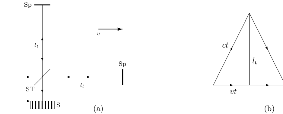
Abbildung 1.1: Das Michelson-Morley-Interferometer. (a) Ein Lichtstrahl trifft auf einen Strahlteiler (ST) und die beiden Anteile breiten sich in orthogonale Richtungen entlang der Strecken l_1 und l_t aus. Sie werden an Spiegeln (Sp) reflektiert, treffen wieder auf den Strahlteiler und können auf dem Schirm (S) interferieren. (b) Der Strahl transversal zur Bewegungsrichtung relativ zum Äther legt die Strecke 2ct zurück, während sich die Apparatur um die Strecke 2vt weiterbewegt hat.
