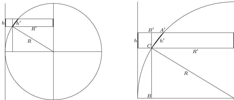
Abbildung 1.9: Zum geometrischen Beweis der Flächentreue der Lambert-Projektion. Die rechte Seite zeigt den Ausschnitt links-oben vergrößert. Da die Strecke A'C senkrecht auf AC steht, sind die Dreiecke ABC und A'B'C ähnlich. Daraus folgt R'/R = h/h' .
