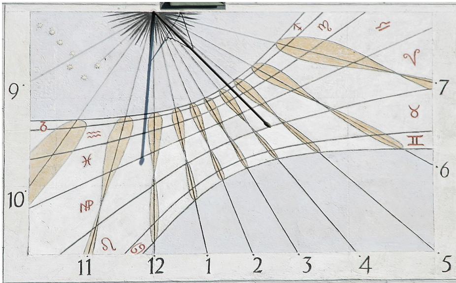
Abbildung 1.1: Sonnenuhr am Alten Rathaus in München. Anhand der Schattenlänge zu verschiedenen Jahreszeiten kann die wahre (angezeigte) Uhrzeit um die Zeitgleichung korrigiert werden, die durch die Analemmas an den Stundenlinien angegeben wird. Die Sternzeichen geben an, welcher Teil des Analemmas (linker oder rechter Rand) in einem bestimmten Monat zu verwenden ist. (aus [1])
