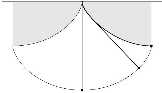
Abbildung 1.6: Die Huygens'sche Aufhängung. Die Cycloide löst gleichzeitig das zweite Problem bezüglich eines von der Auslenkung unabhängigen Pendels: Wenn das schwingende Pendel an seiner Aufhängung durch eine Cycloide begrenzt ist, sodass der obere Teil des Pendelseils an der Cycloide entlang läuft, folgt die Masse am Ende des Pendels einer Cycloide.
